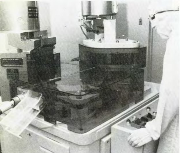
カプセルの充填機
