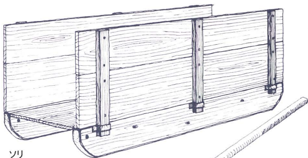
除雪具
