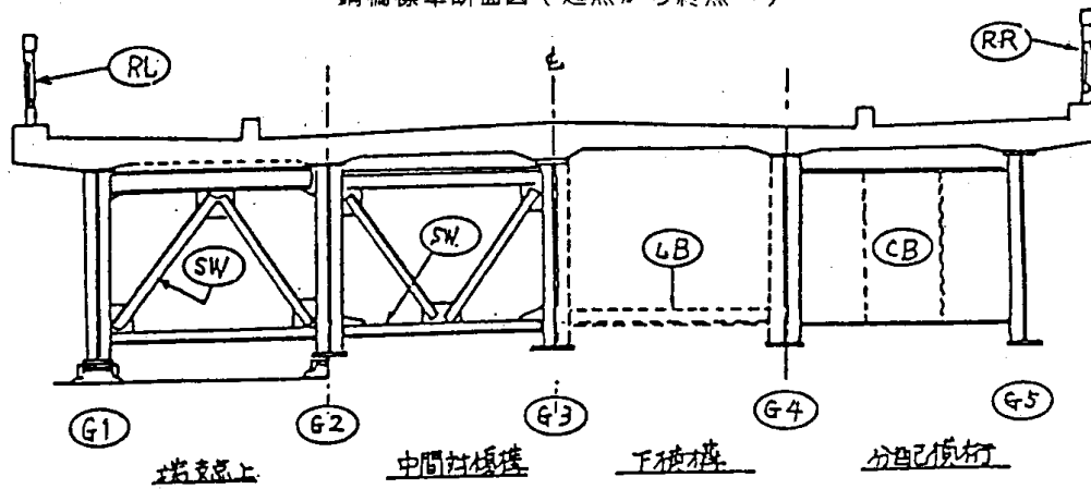
配置図
