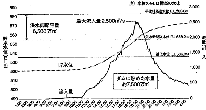
図2 ハツ場ダム地点の洪水ハイドログラフ
