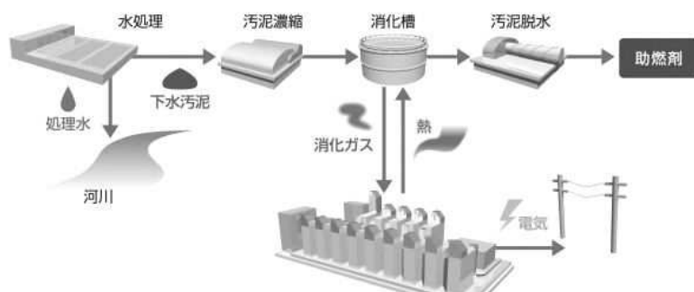
浜黒崎バイオガスパワー 発電のしくみ
