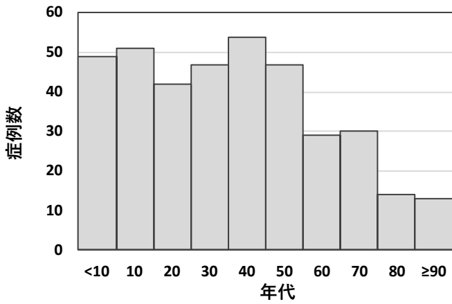
図3. COVID-19年代分布（富山県、11週）
