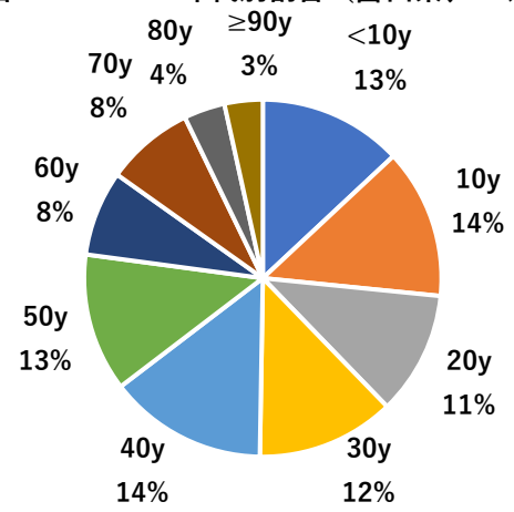
図4. COVID-19年代別割合（富山県、11週）
