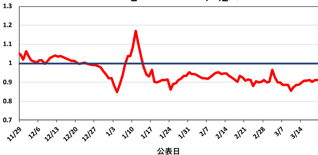
図2. COVID-19_実効再生産数(Rt)_富山県
