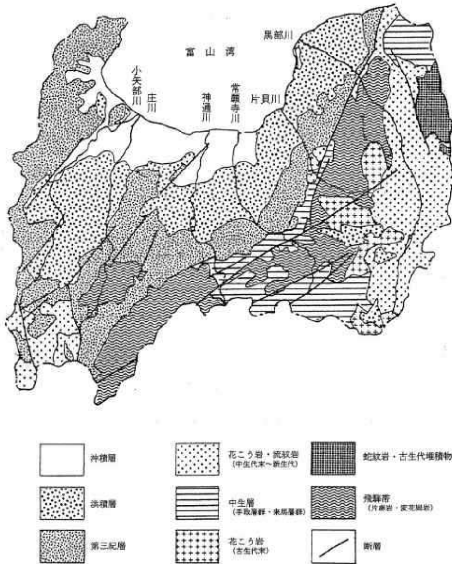
図-1 富山県の地質概要図
