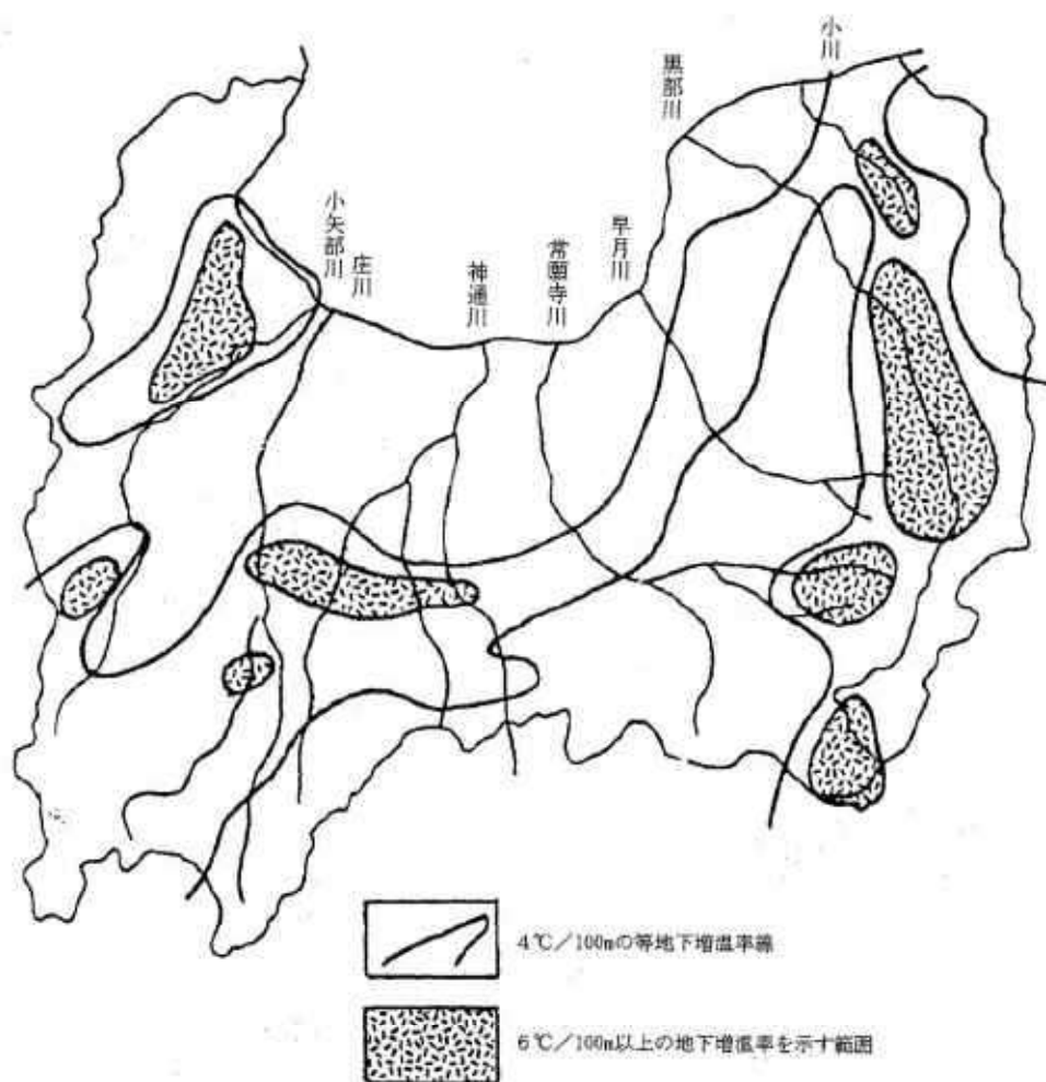
図一 2 富山県内の地熱分布図 富山県（1996）富山県の温泉より
