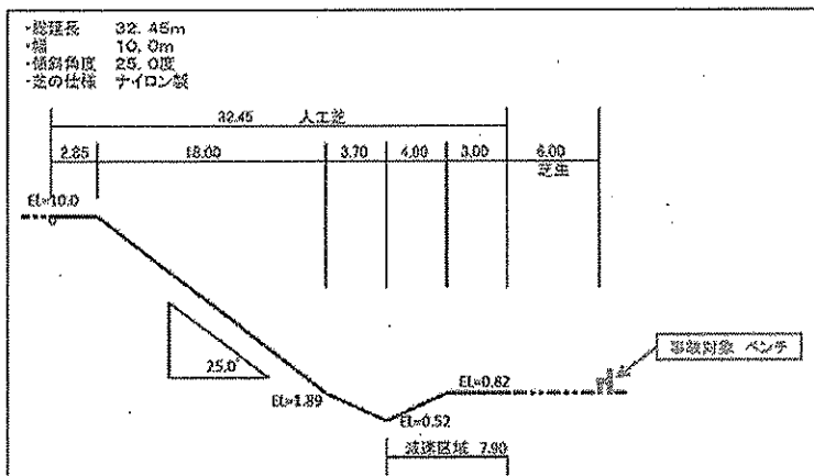
事故が起きた施設の概要図面
