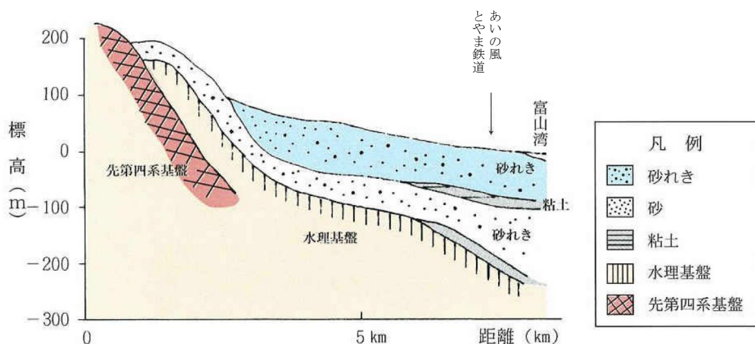
図13 地下地質断面図（魚津・滑川地域）
