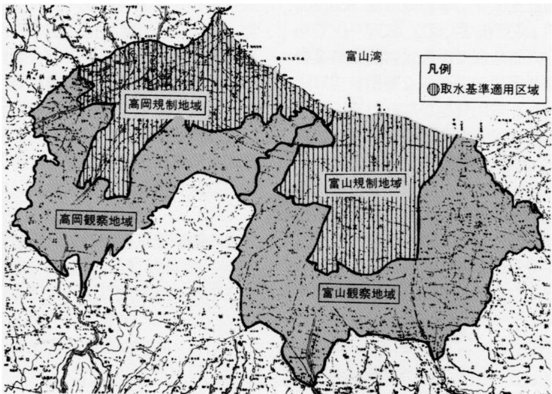
図1 地下水条例指定地域図
