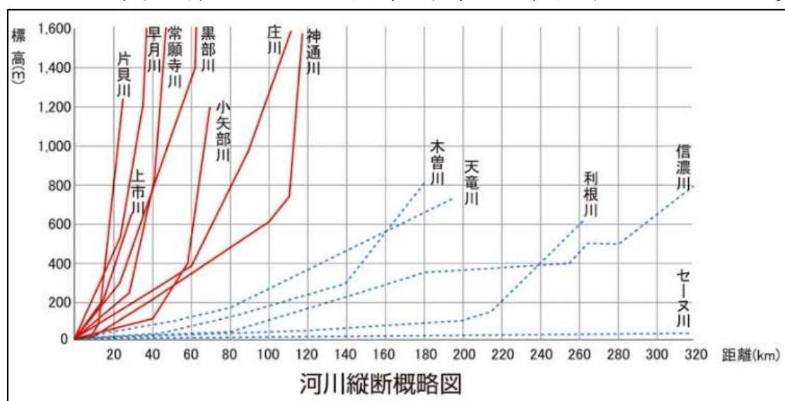
図4 河川縦断図
