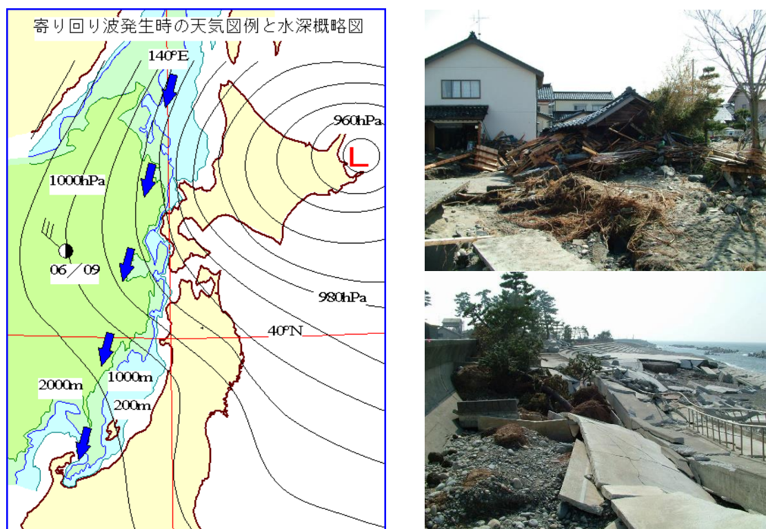
図13 寄り回り波発生時の天気図例と水深概略図と入善町芦崎地区の被害状況
