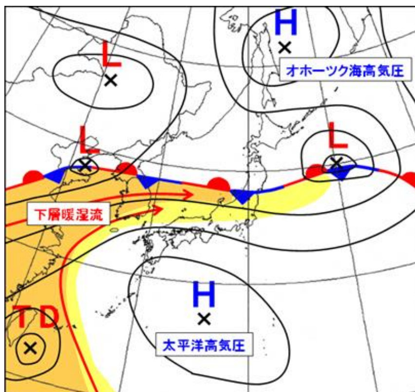
図11 北陸地方で大雨となりやすい天気図（富山地方气象台提供）
