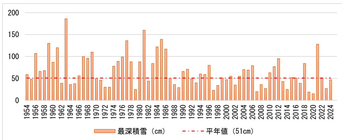
図10 富山市の累年の最深積雪（1954～2024年・寒候期）
