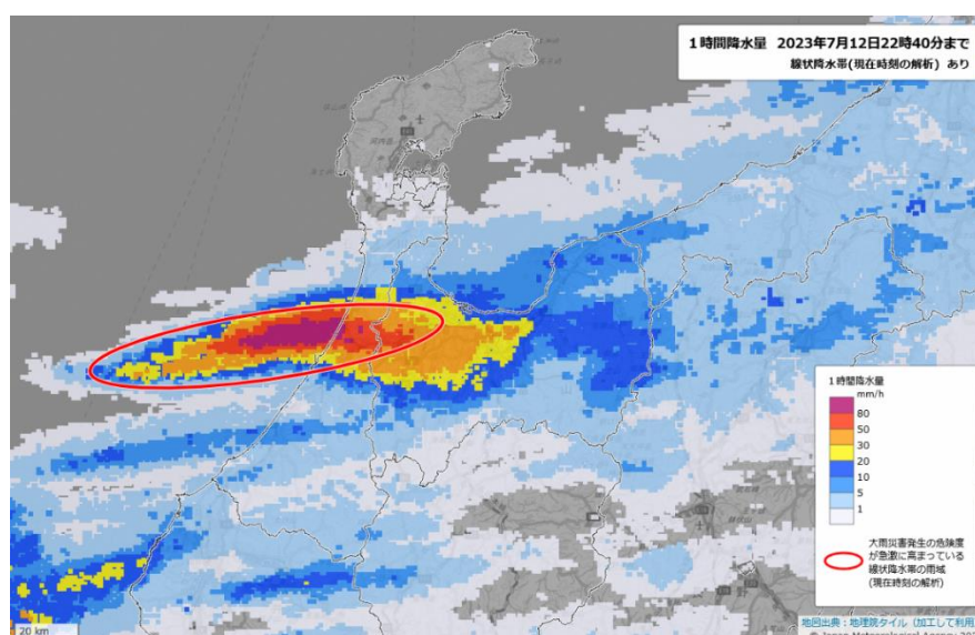
図12 令和5年7月 線状降水帯発生時の「今後の雨」（富山地方气象台提供）
