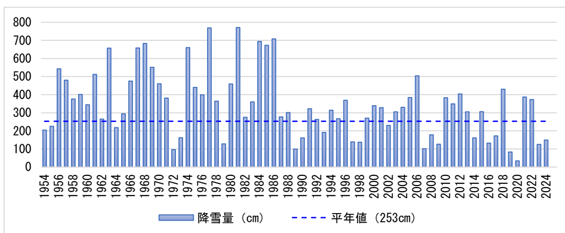
図9 富山市の累年の降雪量（1954～2024年・寒候期）
