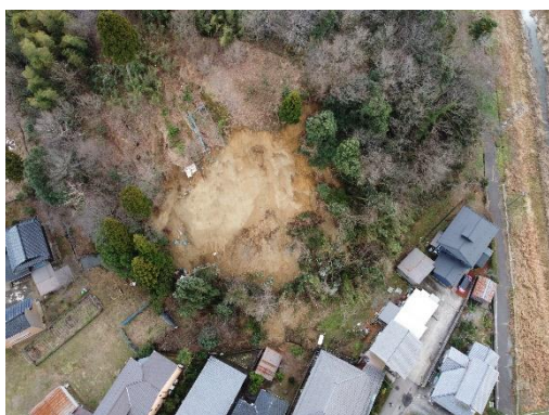
図6 令和6能登半島地震に伴う土砂災害（令和6年1月） （左：氷見市園地内、右：高岡市太田地内）
