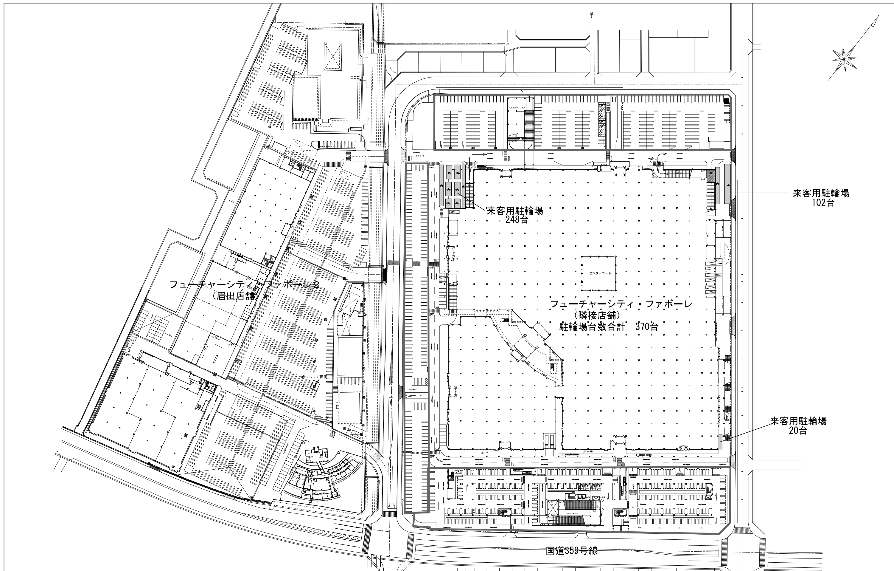
図面 3-1-② 建物配置図【変更前】 (駐輪場図) (S=1/1,600)
