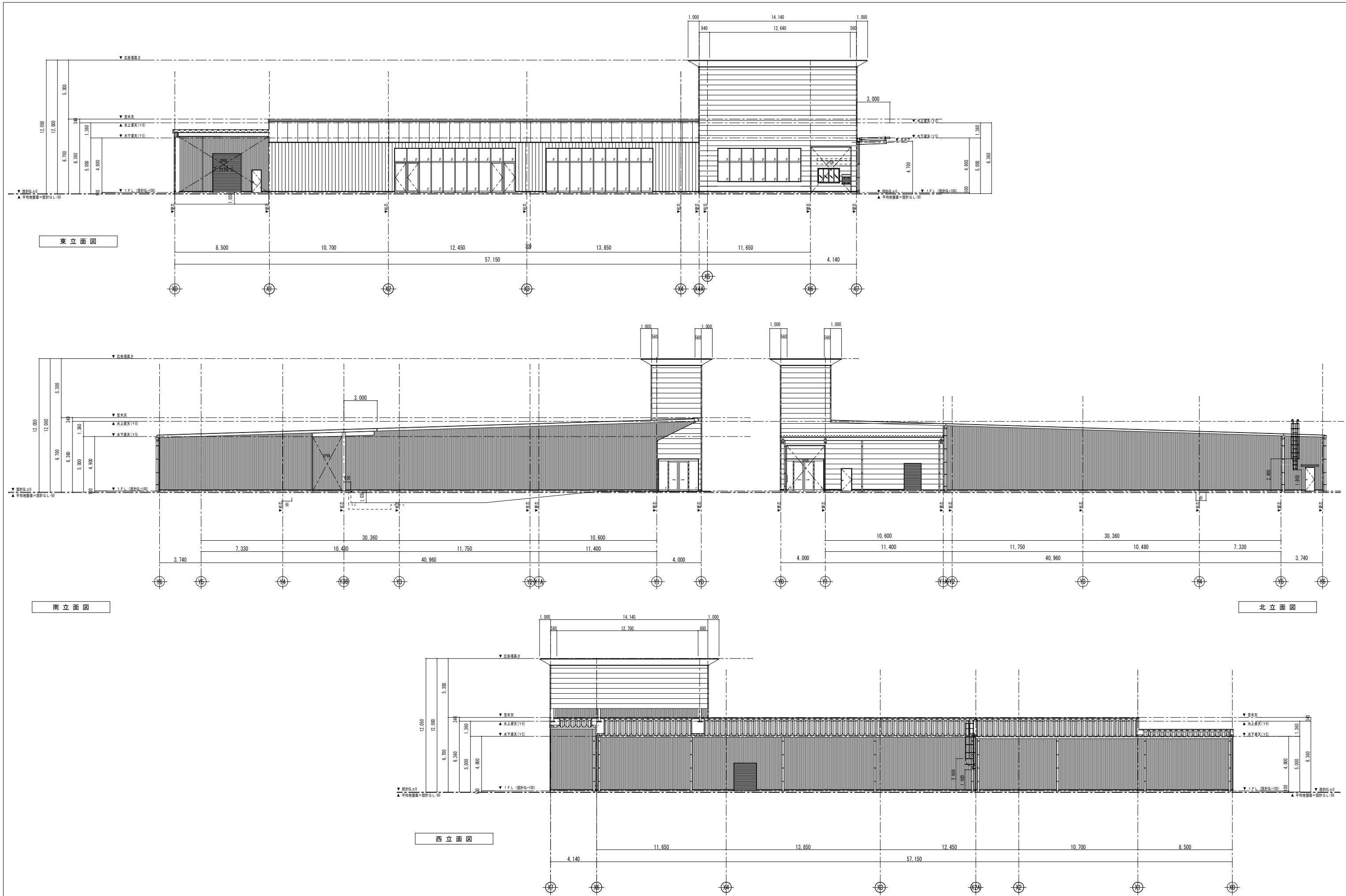
图6 立面图 1/300
