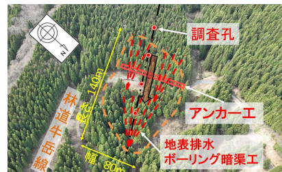
富山市八尾町坂ノ下地区 地すべり防止事業
