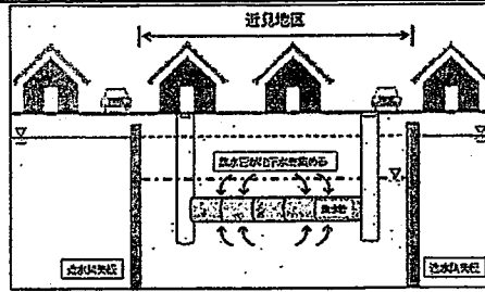
図_地下水位低下工法(イメージ)
