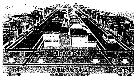
地下水位低下工法
