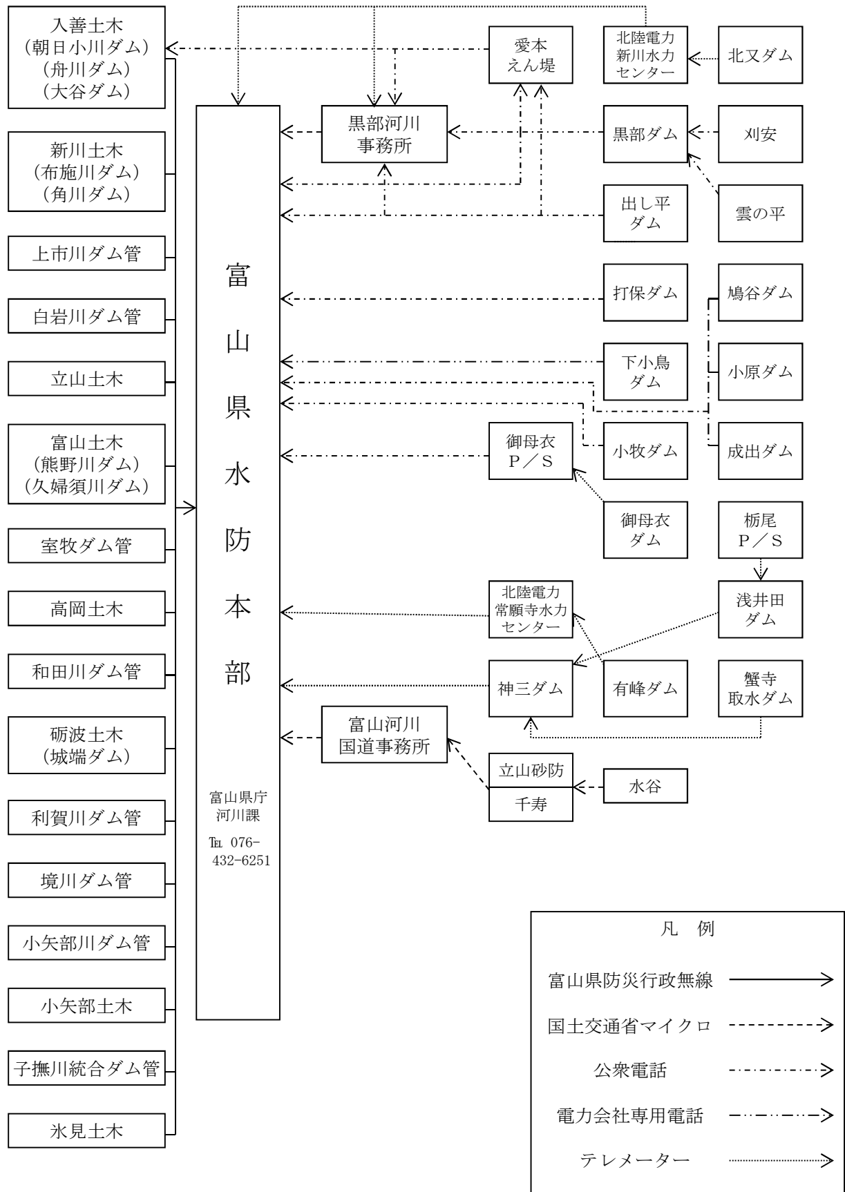
水防本部への雨量通報連絡系統図
