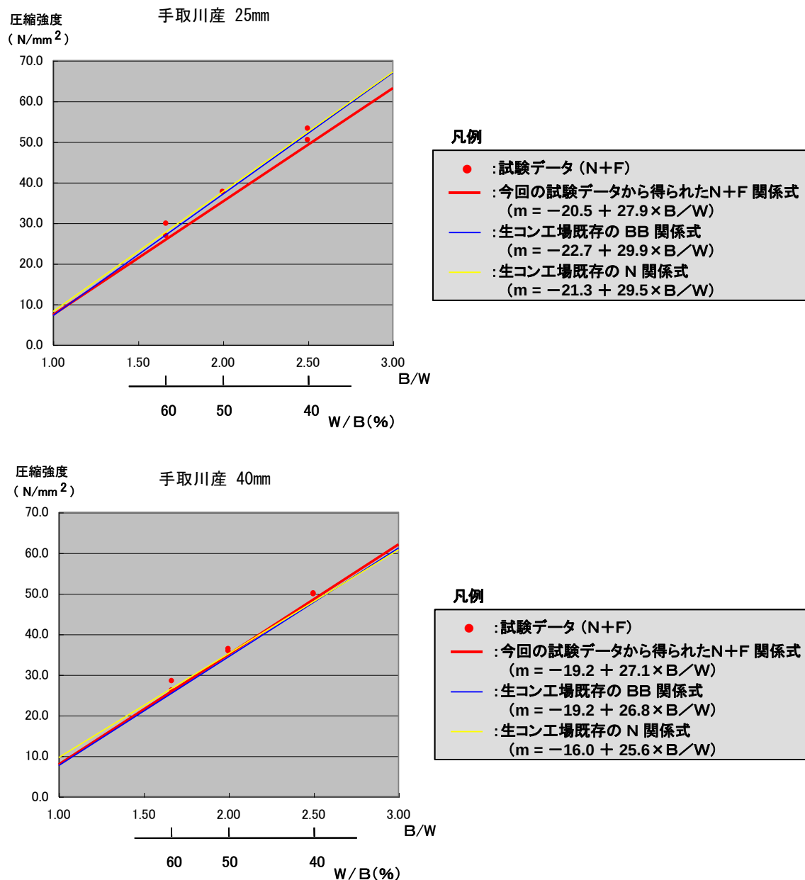
図 3 - 3 手取川産骨材における圧縮強度と結合材水比 (B/W) の関係
