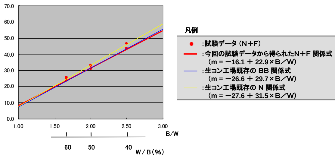
図 3-7 今津産骨材における圧縮強度と結合材水比 (B/W) の関係
