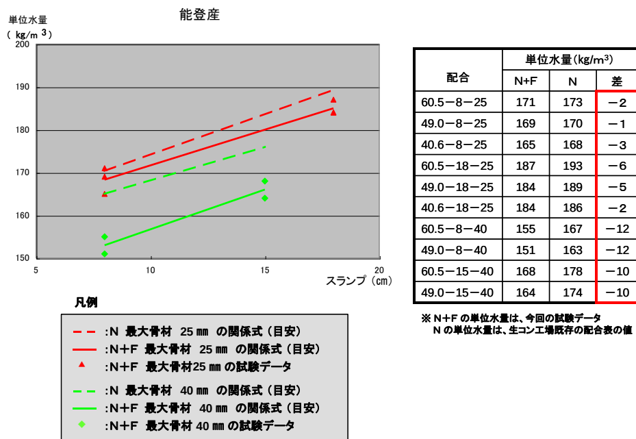
図 3-1-1 能登産骨材におけるスランプと単位水量の関係
