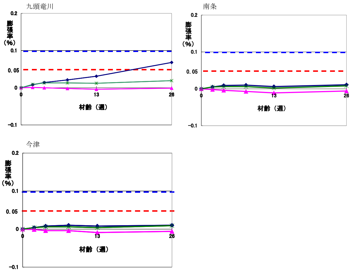
図 2 - 2 モルタルバー法 (JIS A 1146) の結果
