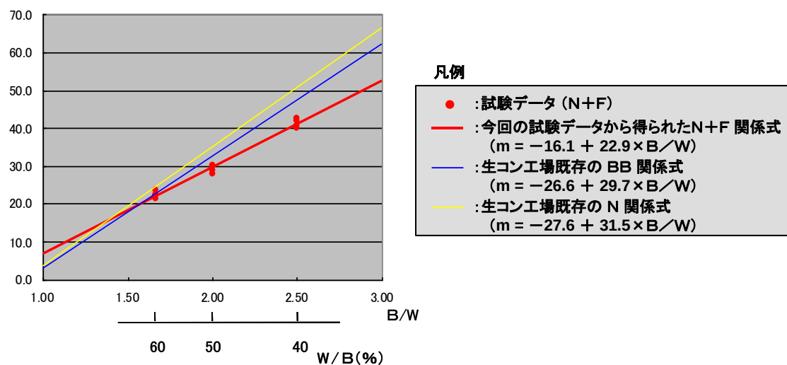
図 3-6 南条産骨材における圧縮強度と結合材水比 (B/W) の関係
