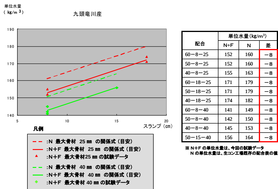
図 3-1-2 九頭竜川産骨材におけるスランプと単位水量の関係
