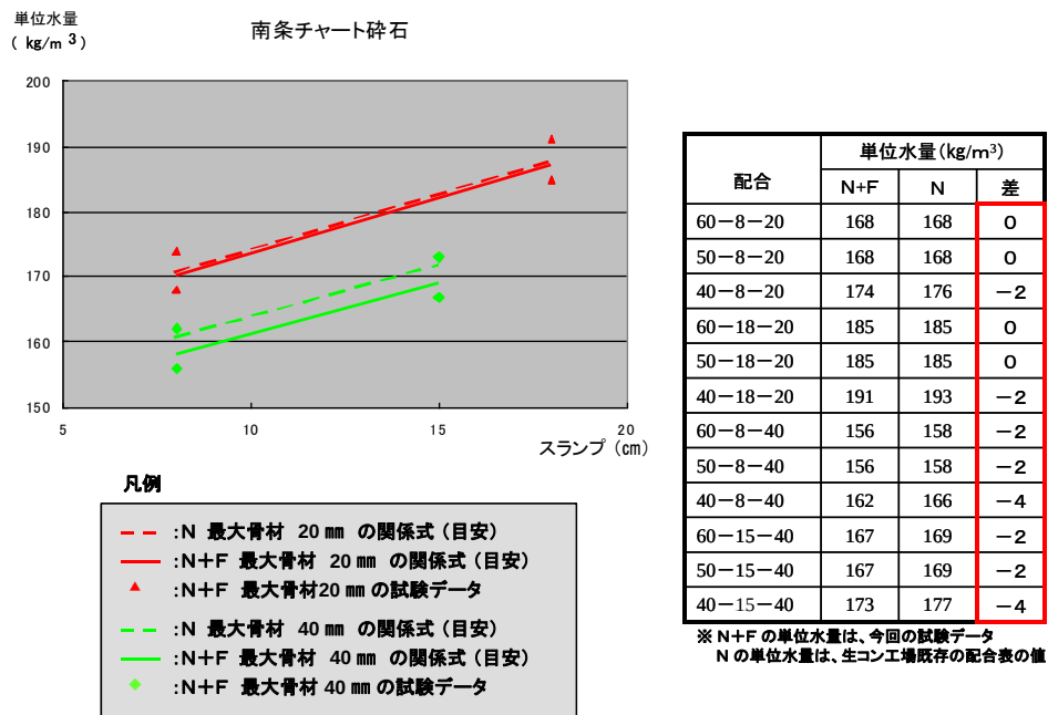
図 3-13 南条産骨材におけるスランプと単位水量の関係
