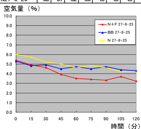
図5-6 早月川産骨材の空気量ロス
