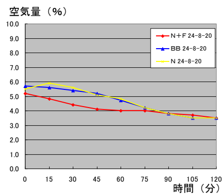
図5-10 南条産骨材の空気量ロス
