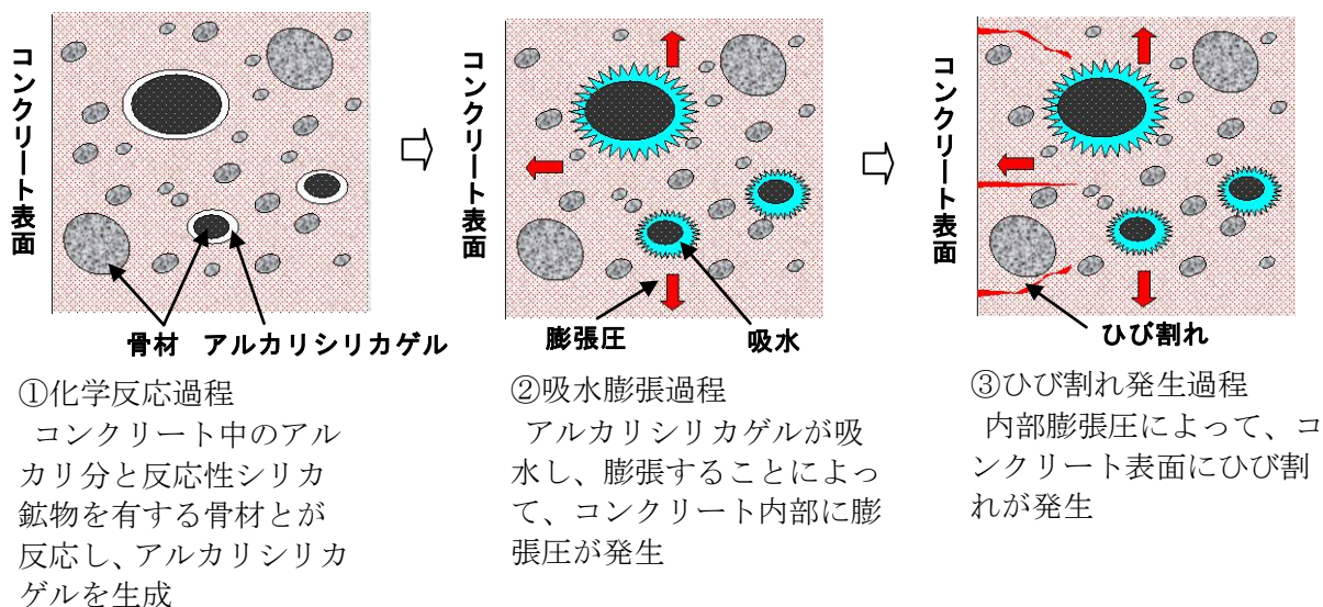
図1-5 アルカリシリカ反応のメカニズム
