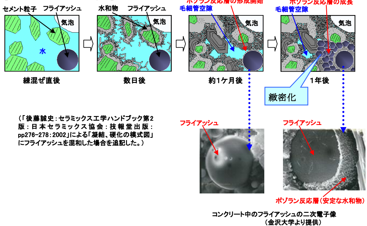
図 1－4 ポズラン反応のメカニズム
