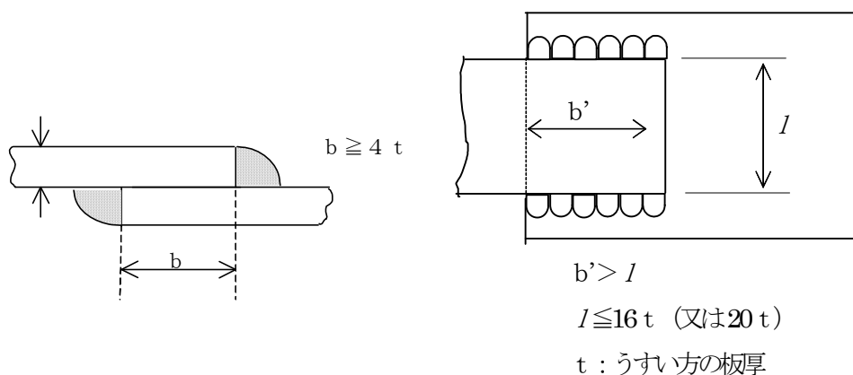
図 11-2-2 前面すみ肉溶接の重ね代 (b)
