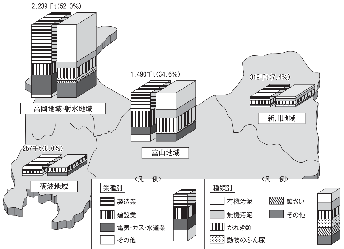
図2-1 産業廃棄物の地域別排出量（23年度）
