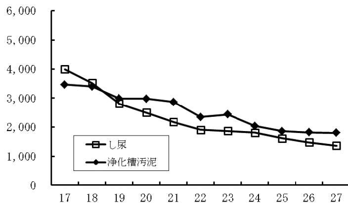
図-11 し尿・浄化槽汚泥処理量の推移（射水市）
