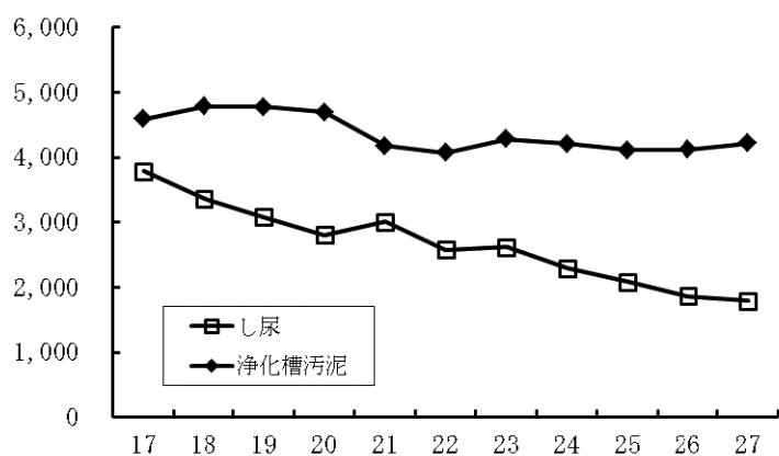
図-9 し尿・浄化槽汚泥処理量の推移（小矢部市）
