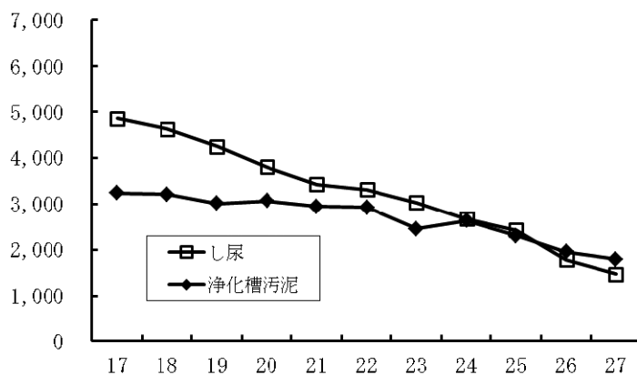
図-13 し尿・浄化槽汚泥処理量の推移（上市町）
