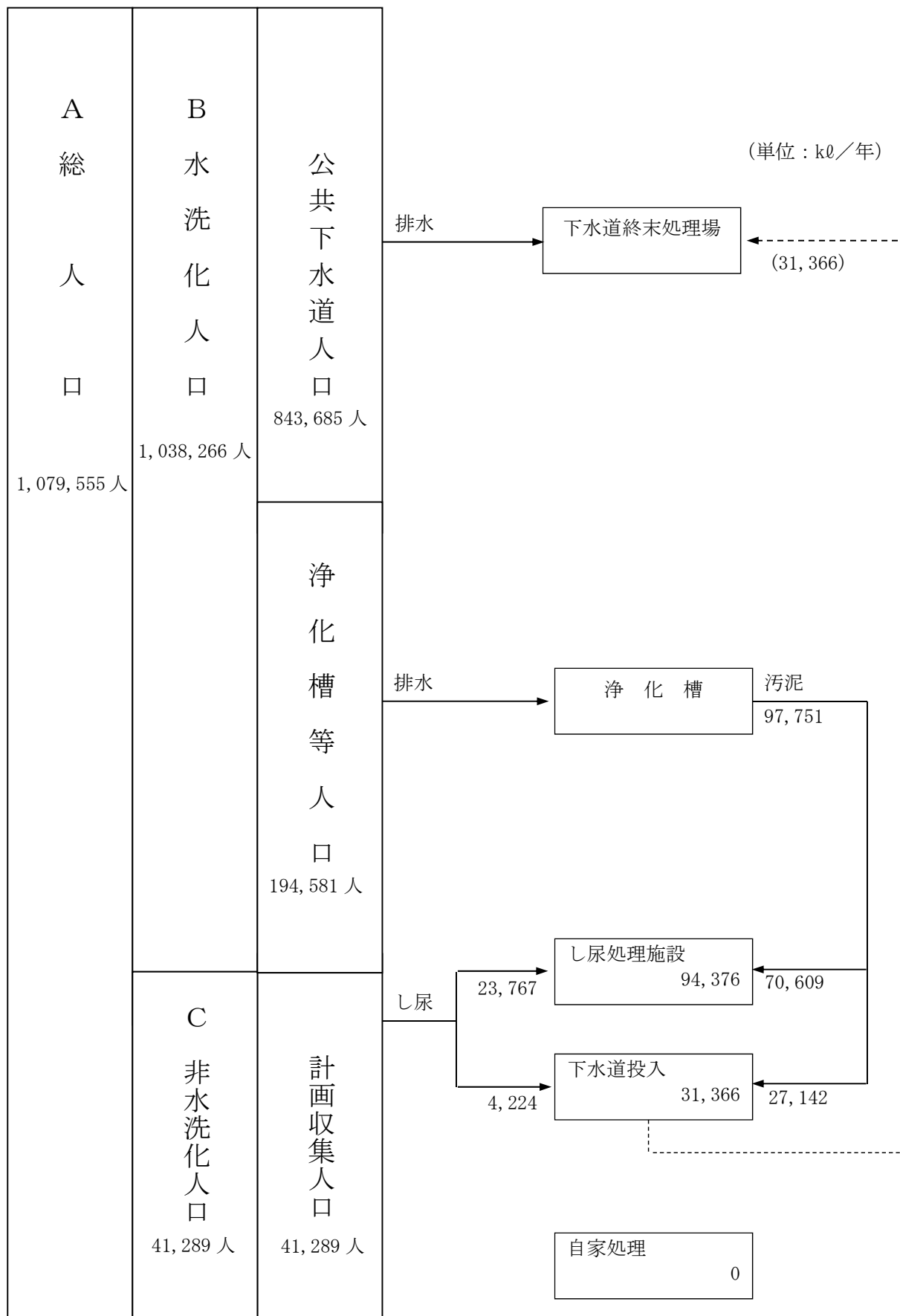
図-8 し尿処理フローチャート(27年度)
