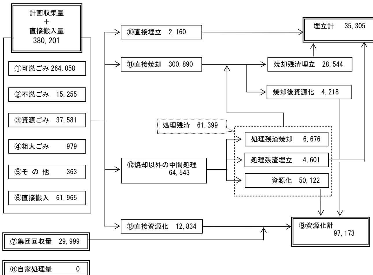
図-4 27年度ごみ処理状況（単位：t）
