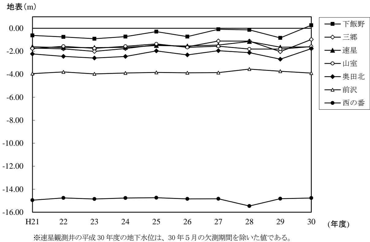
図9-2 地下水位（年平均値）の推移
