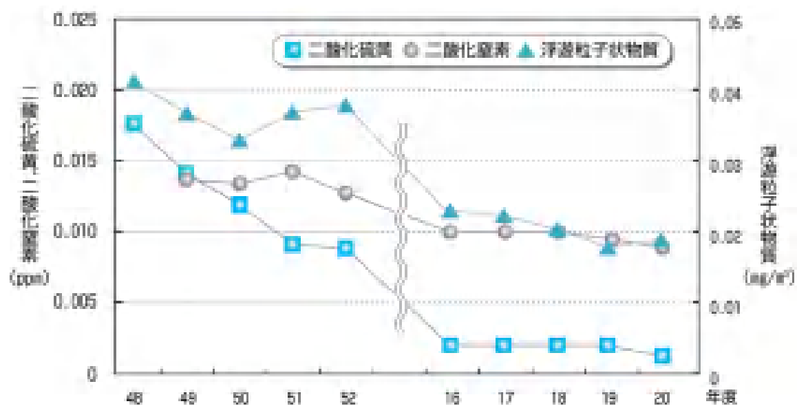
図 1.1.3 主な大気汚染物質の年平均値の推移
