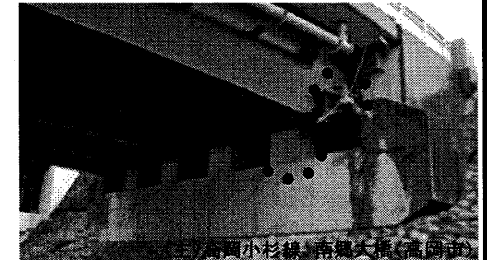
橋梁の耐震化(落橋防止装置設置状況)
