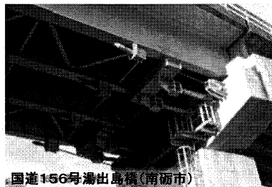
国道156号湯出島橋(南砺市) 橋梁の耐震化(落橋防止装置設置状況)
