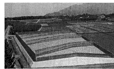
海岸防災林の造成(入善町横山地区)
