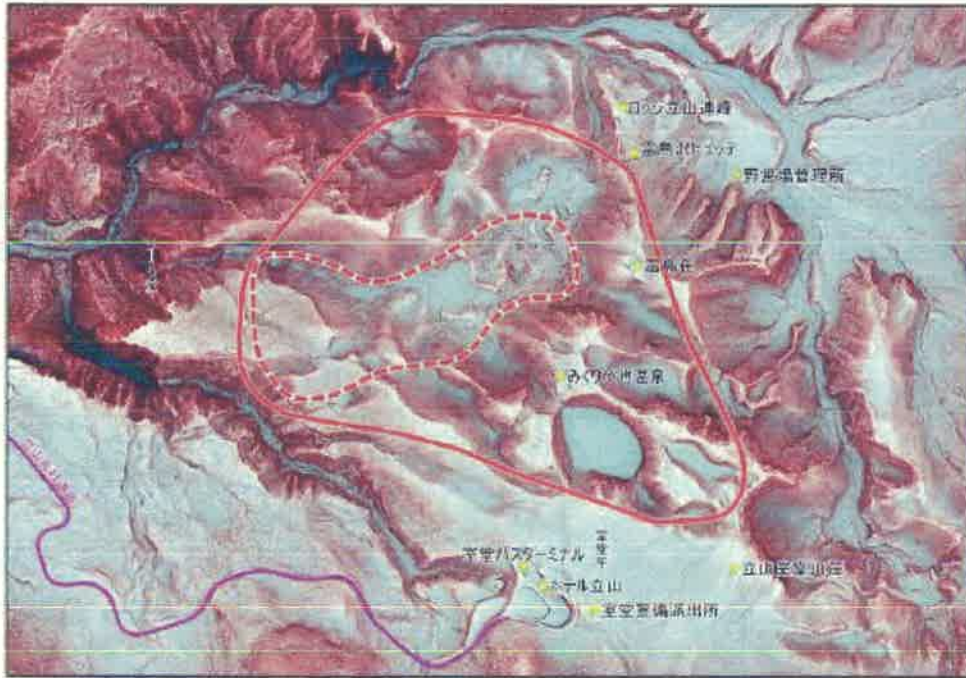
図5 想定火口域
